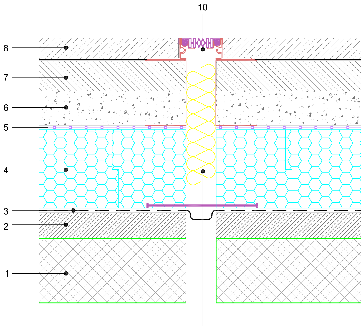
SASTAV SISTEMSKOG RJEŠENJA (dimenzije uskalditi s proračunom građevne fizike):
